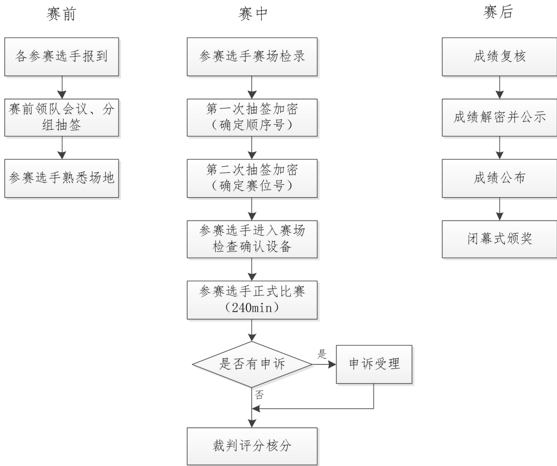
图1 竞赛流程图
